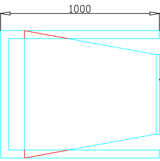
ZIJWAANZICHT
