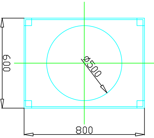
BOVENAANZICHT
